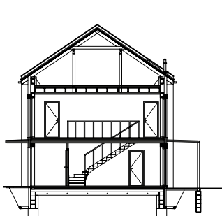
řez
