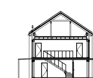
řez
