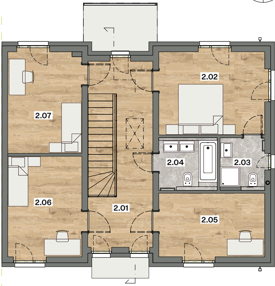
2. NP
