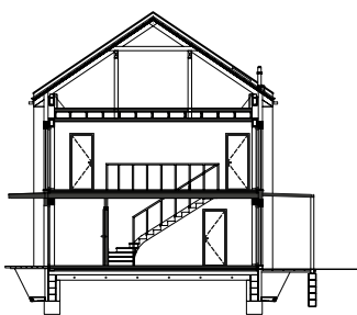
řez
