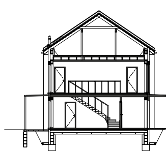
řez
