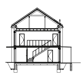
řez
