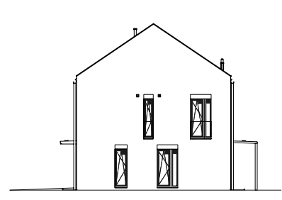
pohled boční
